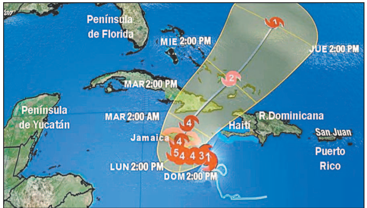
Pronóstico de trayectoria del meteoro desde hoy hasta el jueves de la semana próxima, según el NHC.
