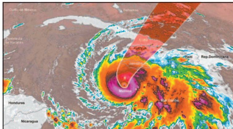
Cono del pronóstico de trayectoria para hoy y los días siguientes.
