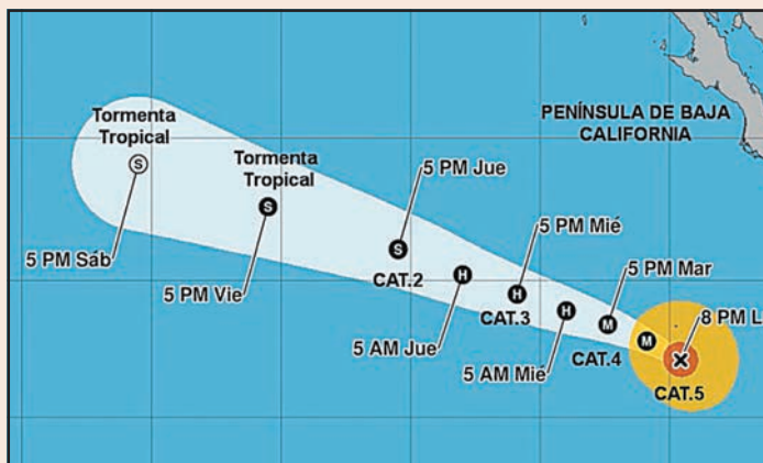
El fenómeno atmosférico se degradará de forma progresiva.
